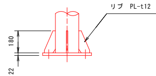
ベースプレート詳細図 S=1:15
